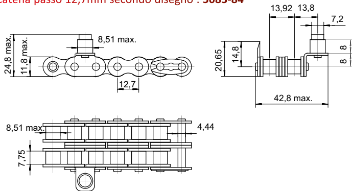
Catena passo 12,7mm secondo disegno : 5083-84
