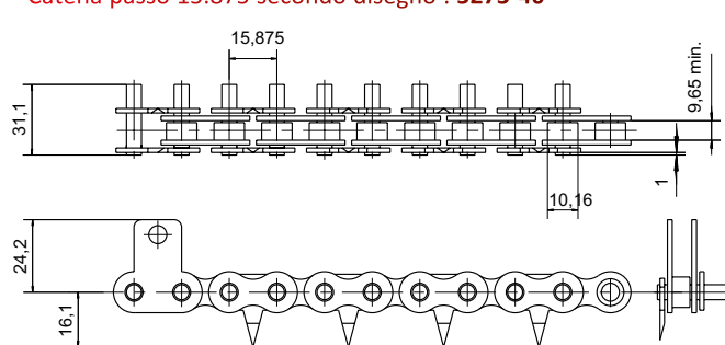
Catena passo 15.875 secondo disegno : 5273-40
